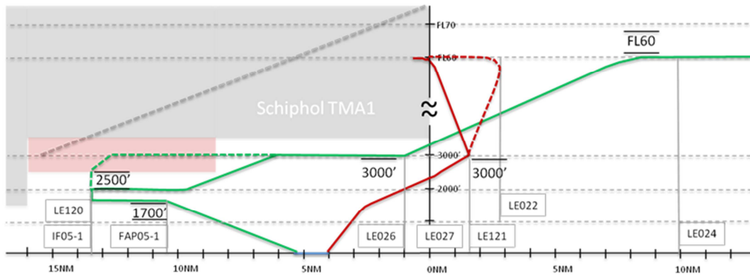
Figuur 64 – Projectie route A baan 05
