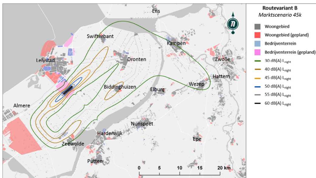
Figuur 43 - Geluidscontouren L_{night} Variant B 45k marktscenario
