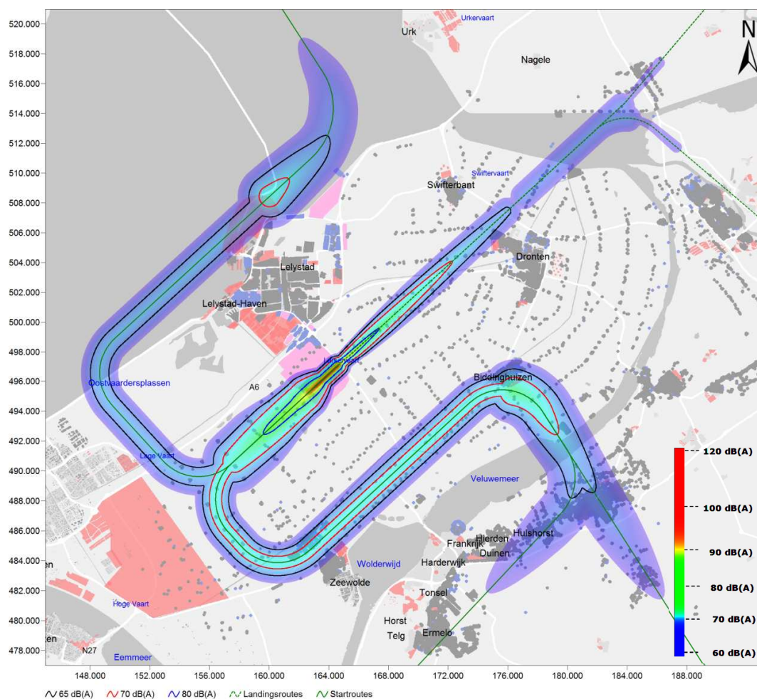
Figuur 49 LA_{max} van een B737-800 voor routevariant A, in het geval baan 23 in gebruik is. (start richting zuidwesten en landing vanuit noordoosten)
