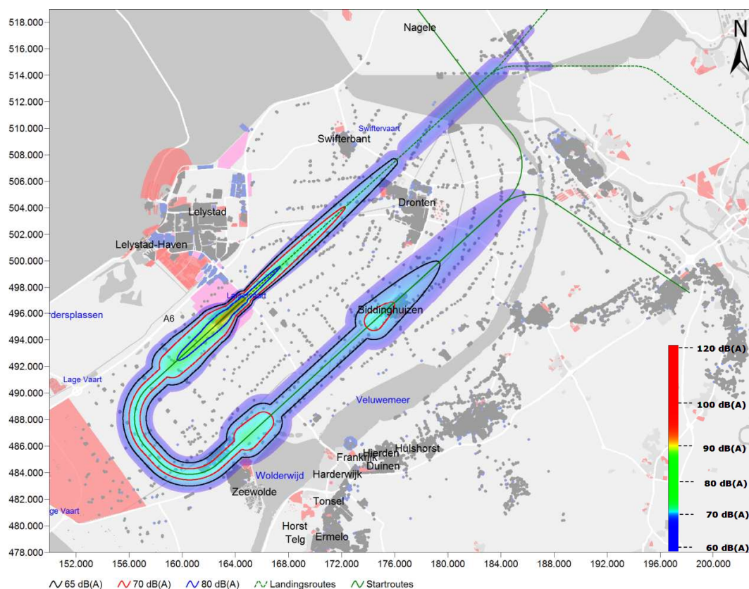
Figuur 51 LA_{max} van een B737-800 voor routevariant B, in het geval baan 23 in gebruik is. (start richting zuidwesten en landing vanuit noordoosten)
