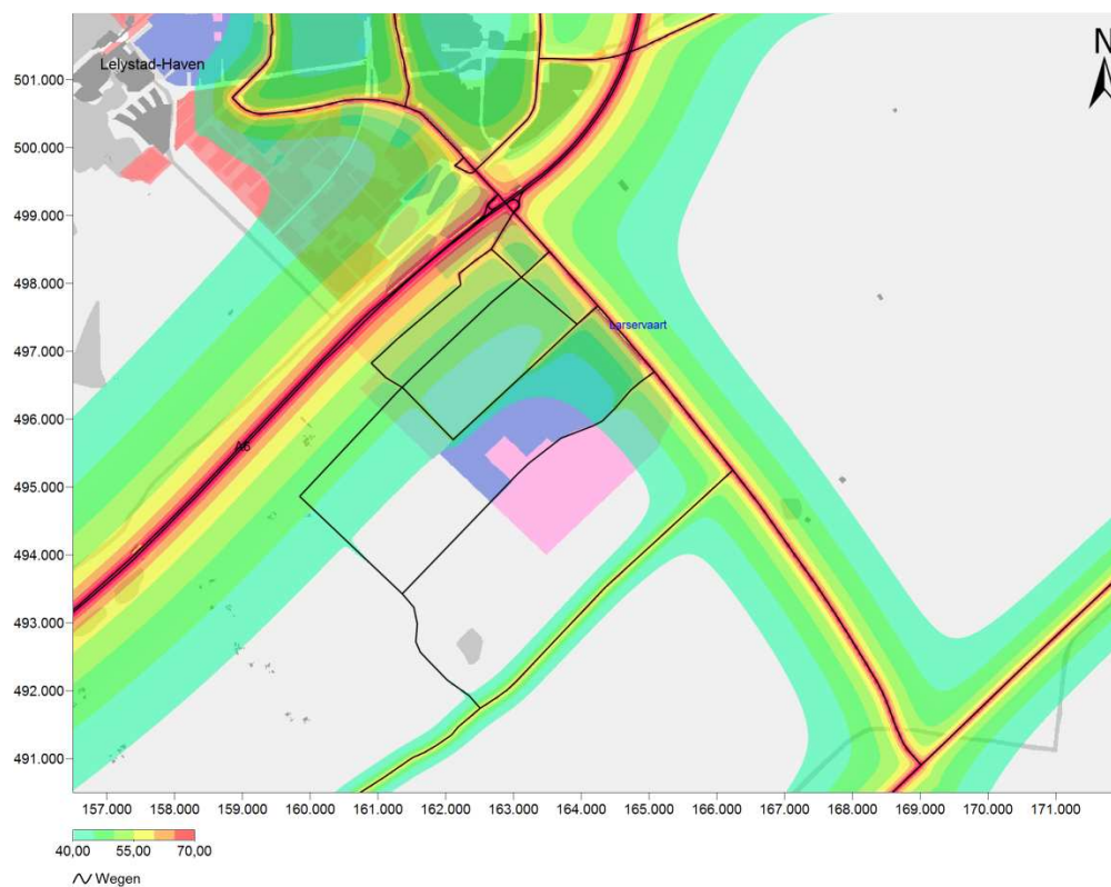
Figuur 56 Geluidbelasting van het wegverkeer in L den voor de autonome ontwikkeling 2025.
