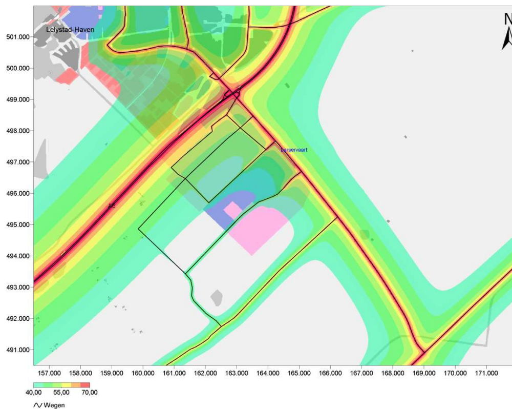
Figuur 58 Geluidbelasting van het wegverkeer in L_{den} voor de voorgenoemde activiteit 2025 (marktscenario 45k).
