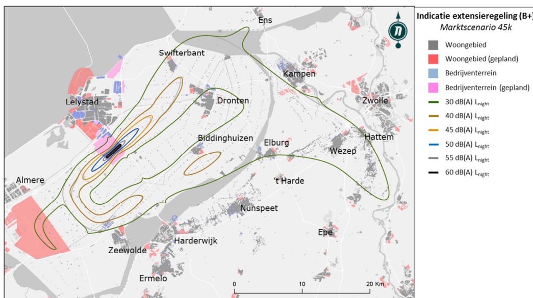
Figuur 46 – Indicatie van het effect van de extensieregeling op L_{night} geluidsbelasting
