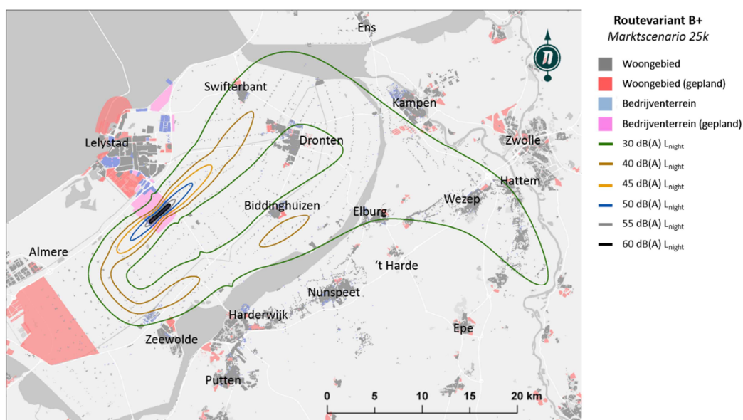
Figuur 44 – Geluidscontouren L_{\text{night}} Variant B+ 25k marktscenario
