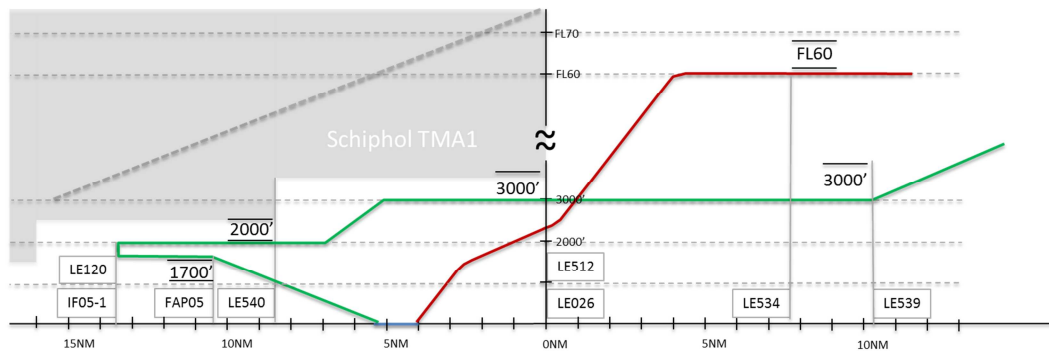
Figuur 67 – Projectie route B baan 05
