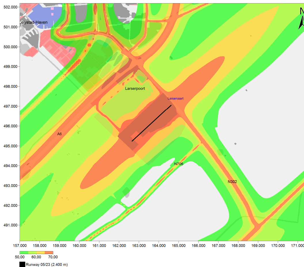
Figuur 62 Cumulatie van geluid in dB(A) L_{den} voor de voorgenomen activiteit (45k) inclusief een extra aansluiting van de A6 naar Lelystad
