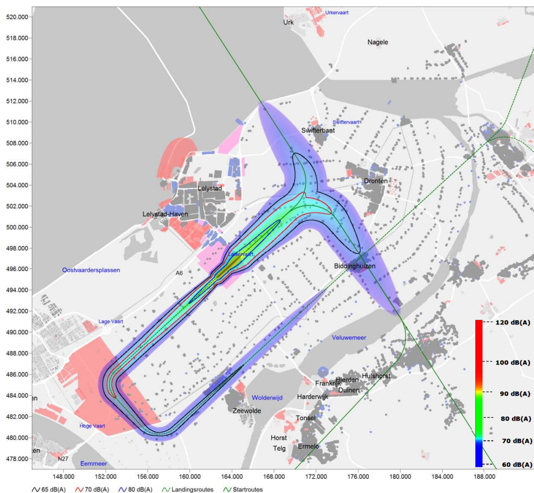
Figuur 48 LA_{max} van een B737-800 voor routevariant A, in het geval baan 05 in gebruik is. (start richting noordoosten en landing vanuit zuidwesten)
