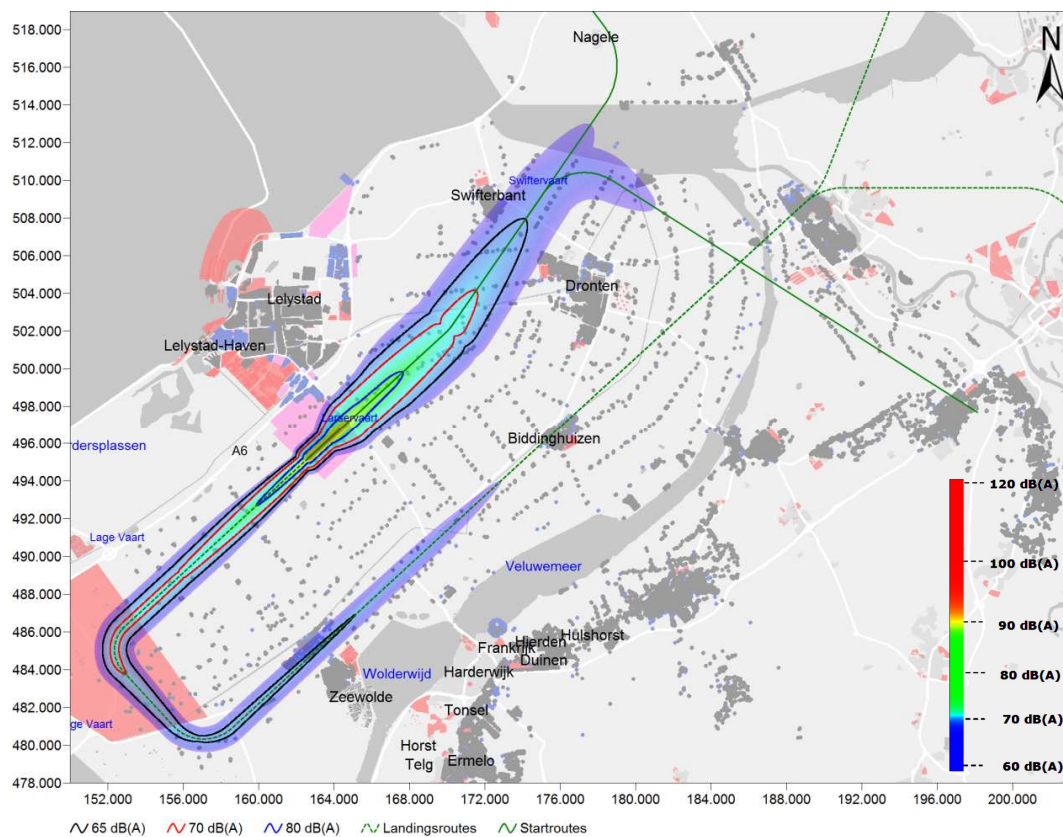
Figuur 50 LA_{max} van een B737-800 voor routevariant B, in het geval baan 05 in gebruik is. (start richting noordoosten en landing vanuit zuidwesten)
