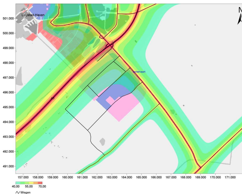
Figuur 54 Geluidbelasting van het wegverkeer in L_{den} voor de autonome ontwikkeling 2015.
