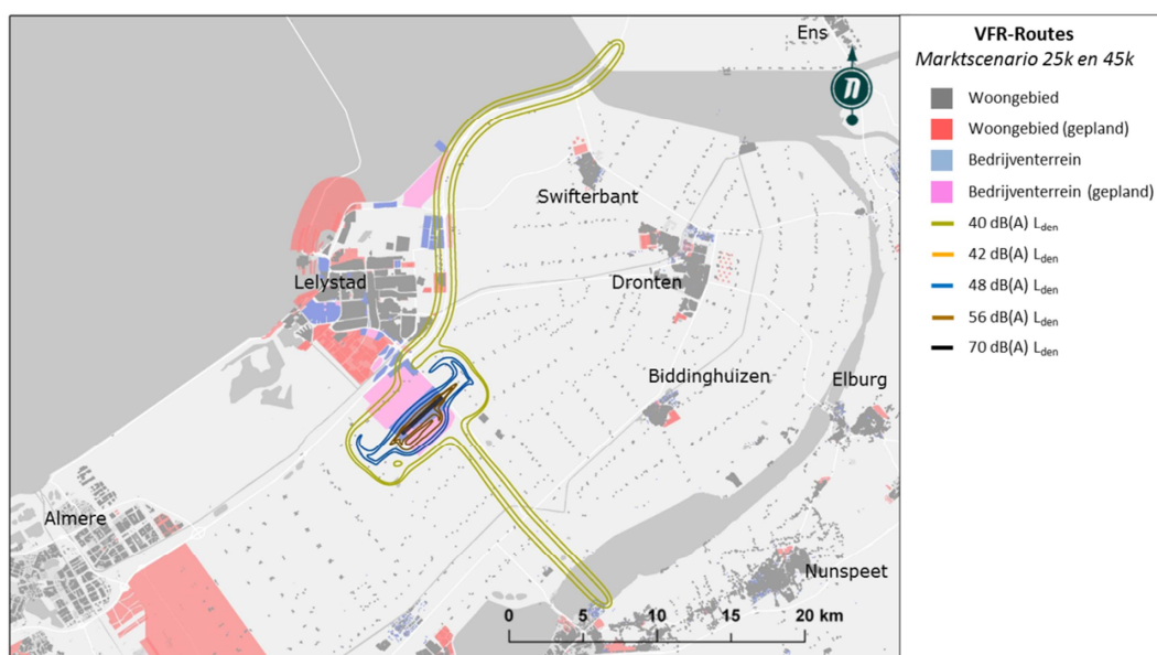
Figuur 38 - Geluidscontouren L_{den} VFR 25k en 45k marktscenario
