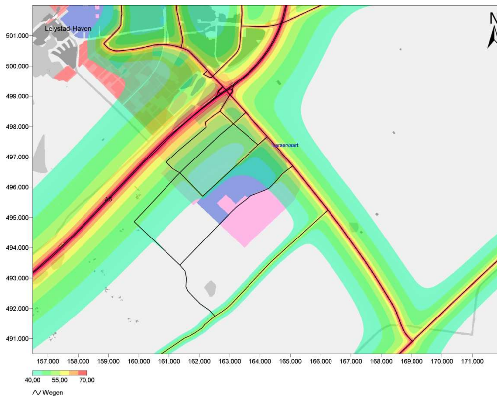
Figuur 55 Geluidbelasting van het wegverkeer in L den voor de autonome ontwikkeling 2020.
