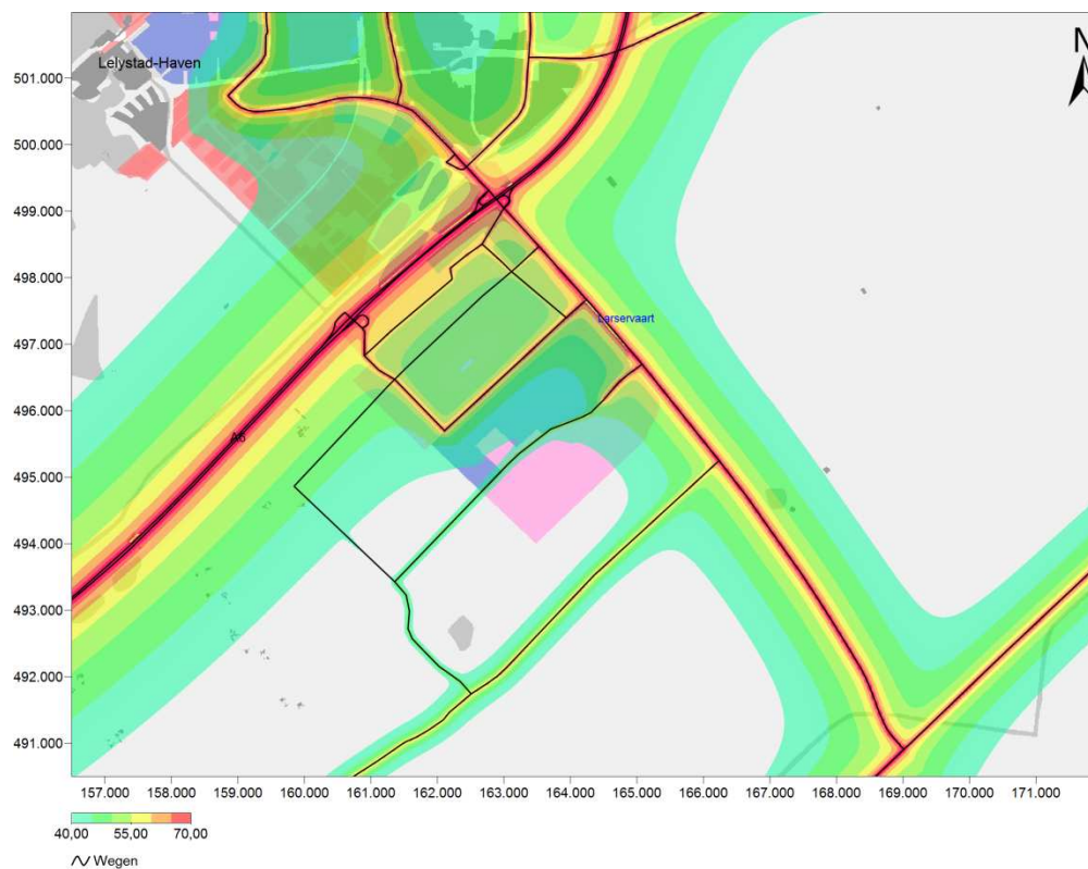
Figuur 59 Geluidbelasting van het wegverkeer in L_{den} voor de voorgenomen activiteit 2025 (marktsценario 45k), waarbij er een 3 e aansluiting op de snelweg A6 is opgenomen.
