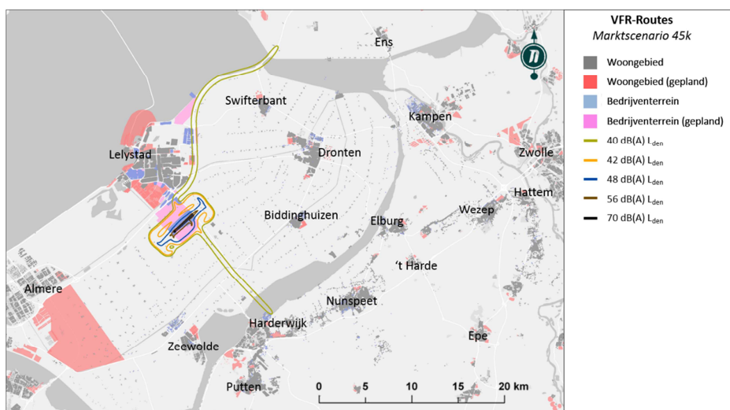
Figuur 36 – Geluidscontouren voor alleen het klein verkeer bij 45 k.
