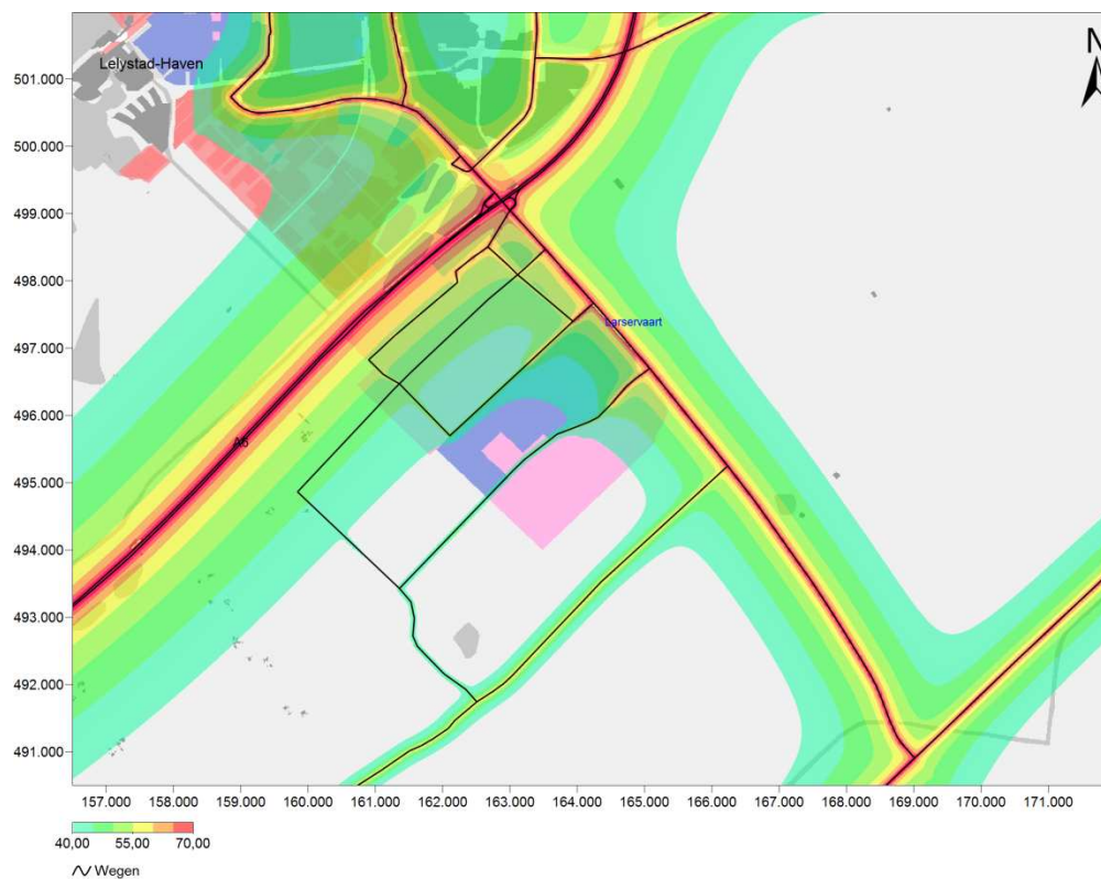
Figuur 57 Geluidbelasting van het wegverkeer in L_{den} voor de voorgenoemde activiteit 2020 (marktscenario 25k).
