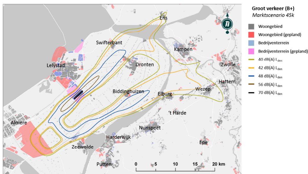
Figuur 37 - Geluidscontouren voor alleen het groot verkeer bij 45 k voor B+
