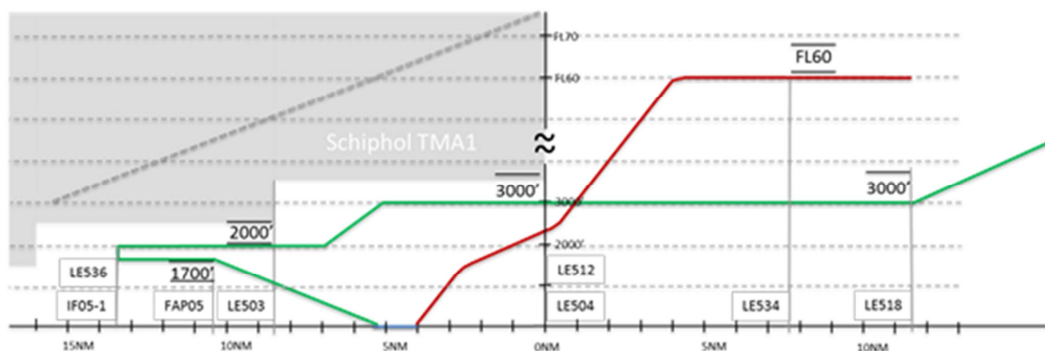
Figuur 70 – Projectie route B+ baan 05
