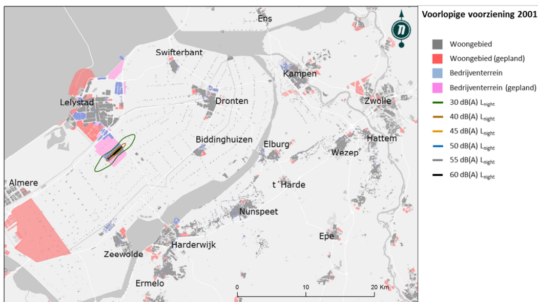
Figuur 39 - 30 t/m 60 L_{\text{night}} -contouren van voorlopige voorziening (Aanwijzing 2001).
