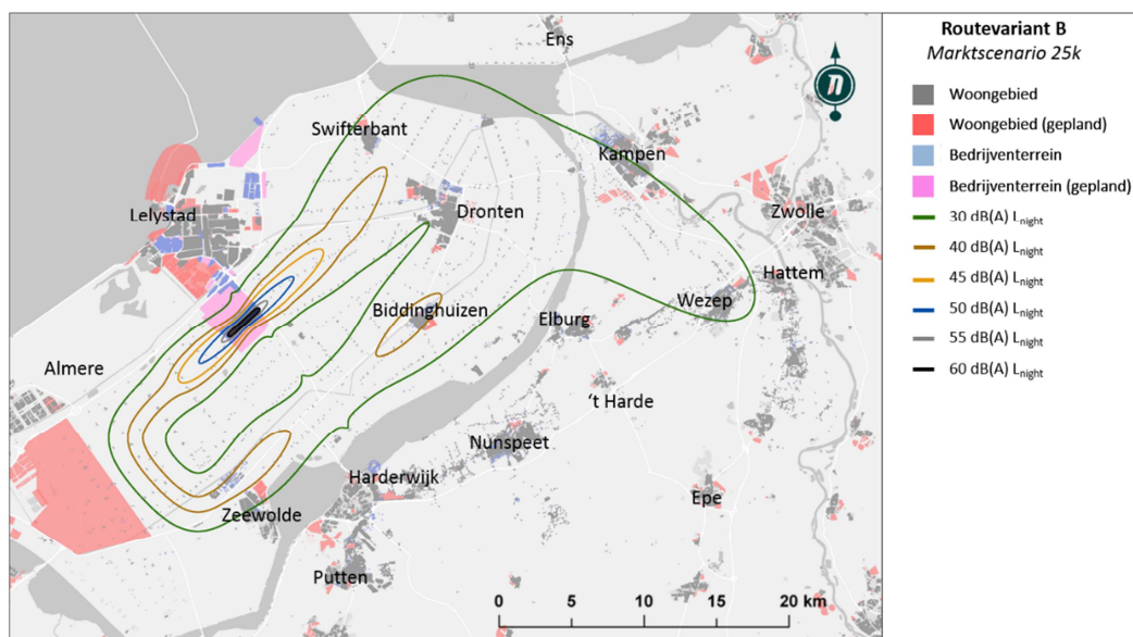
Figuur 42 - Geluidscontouren L_{night} Variant B 25k marktscenario
