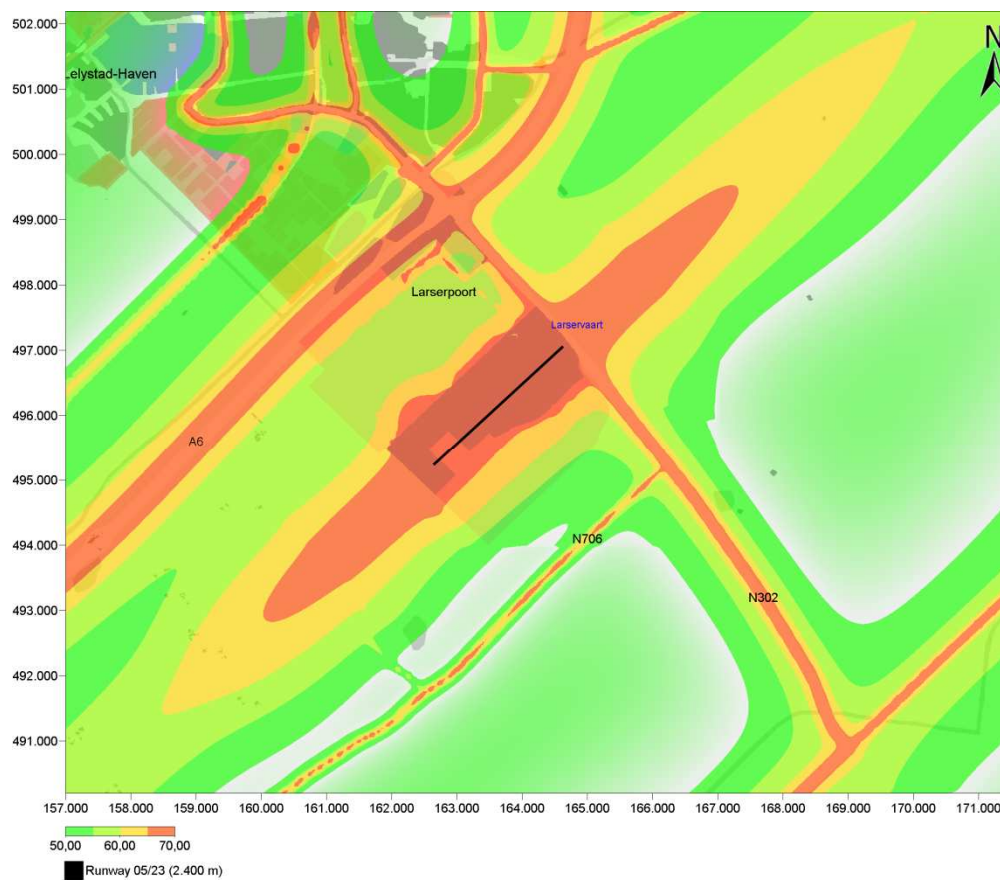
Figuur 61 Cumulatie van geluid in dB(A) L den voor de voorgenomen activiteit (45k).
