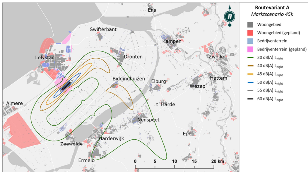
Figuur 41 - Geluidscontouren L_{night} Variant A 45k marktscenario
