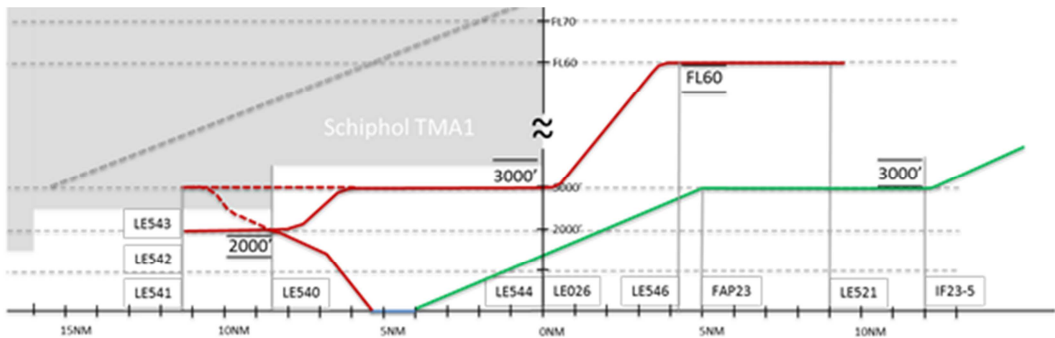
Figuur 65 – Projectie route A+ baan 23
