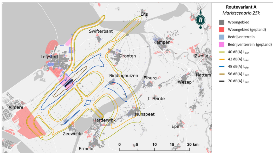
Figuur 23 – Geluidscontouren L_{den} Variant A 25k marktscenario
