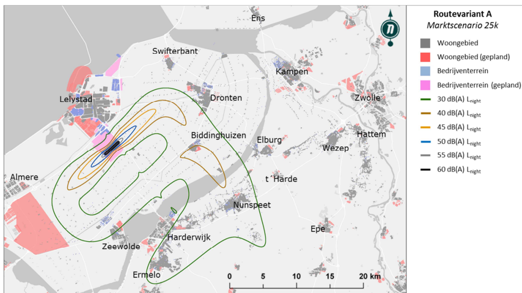
Figuur 40 – Geluidscontouren L_{night} Variant A 25k marktscenario
