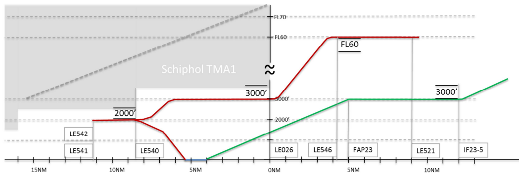
Figuur 68 – Projectie route B baan 23
