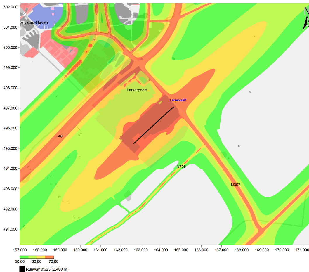
Figuur 60 Cumulatie van geluid in dB(A) L_{den} voor de voorgenoemen activiteit (25k).
