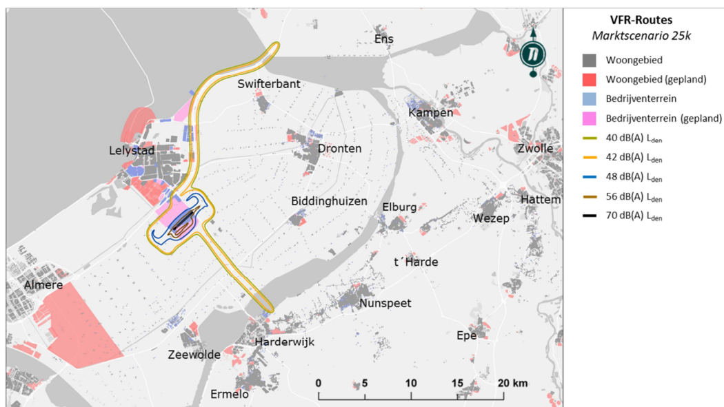
Figuur 35 – Geluidscontouren voor alleen het klein verkeer bij 25 k.
